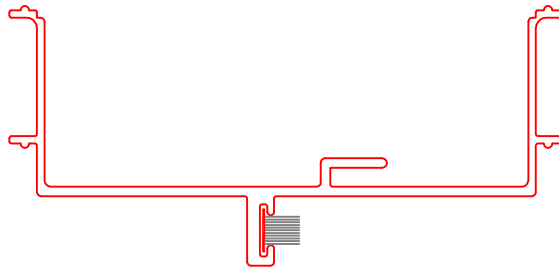
CW 93-9-1 ADF HEADER DRYWALL
